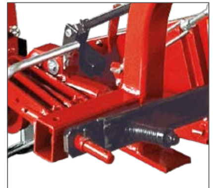
Dispositivo di sicurezza in caso di urti Safety device in case of collisions
